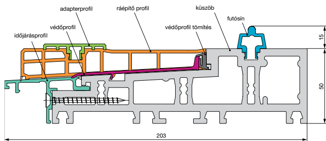
Thermo Top 2.1 küszöb 79 - 92 mm ajtóvastagsághoz.
