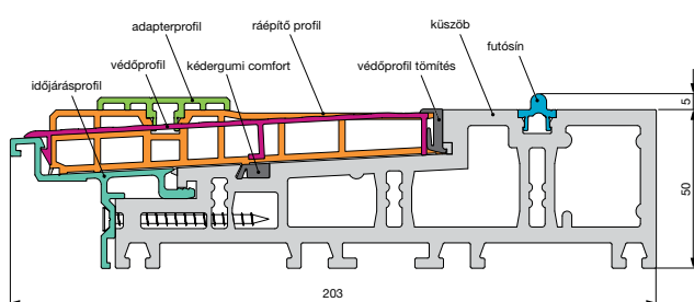
Thermo Top 2.1 comfort padlóküszöb 79 - 92 mm ajtóvastagsághoz.
