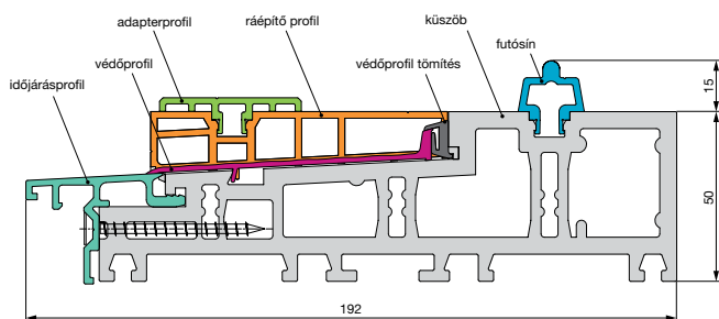
Thermo Top 2.1 küszöb 68 - 78 mm ajtóvastagsághoz.
