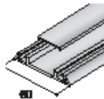
Profil S66NH tárcsaprofil S66N
