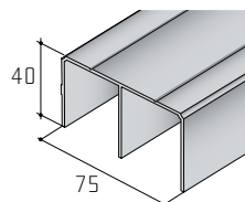
Felső futósín S05
