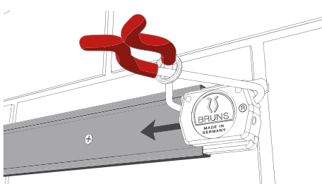
Összeszerelés, 2. lépés
