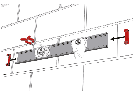
Összeszerelés, 4. lépés
